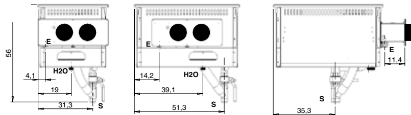
Elektro-Nudelkocher, 42 L
