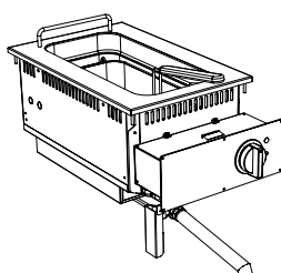
Elektro-Fritteuse, 15 Liter
